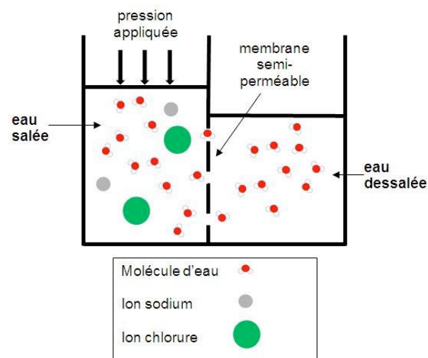
Schéma d'un osmoseur
