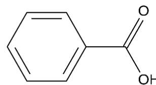
Formule topologique de l'acide benzoïque
