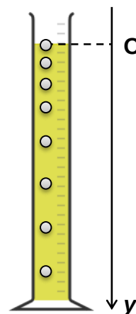
Chronophotographie de la chute de la bille
