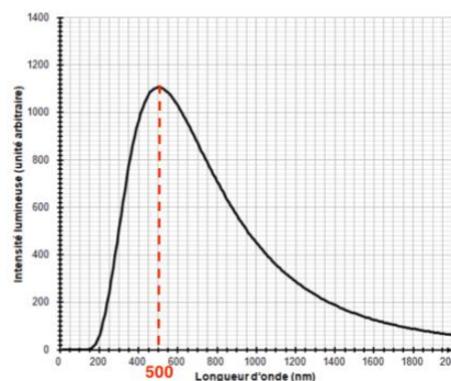
Document 2- Spectre d'émission du Soleil
