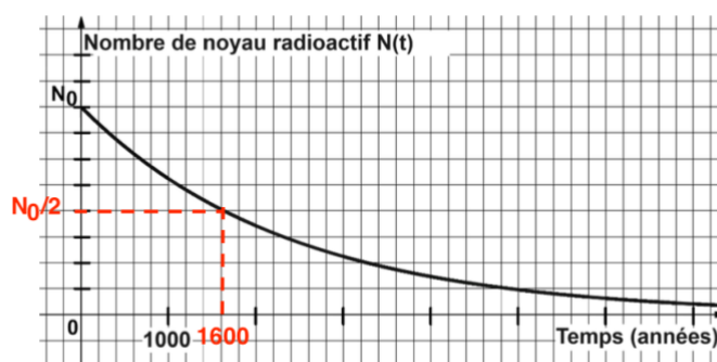
Document 1 – Décroissance radioactive du radium
