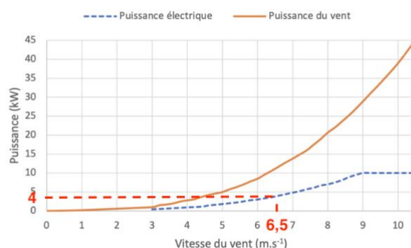
Document 2 – Graphique présentant la puissance électrique réellement produite par l'éolienne et celle du vent, chacune en fonction de la vitesse du vent
