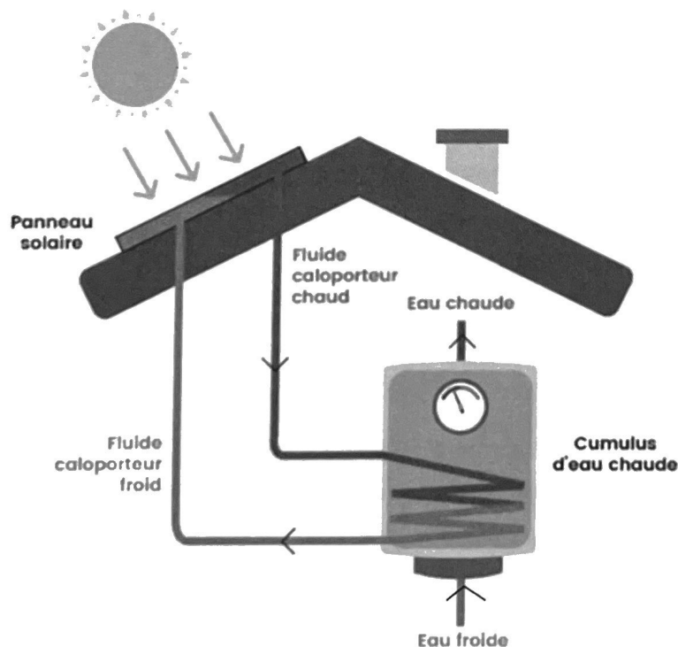
Figure 1 : Schéma du dispositif
