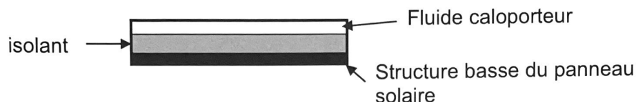
Figure 2 : Schéma de la structure du panneau solaire
