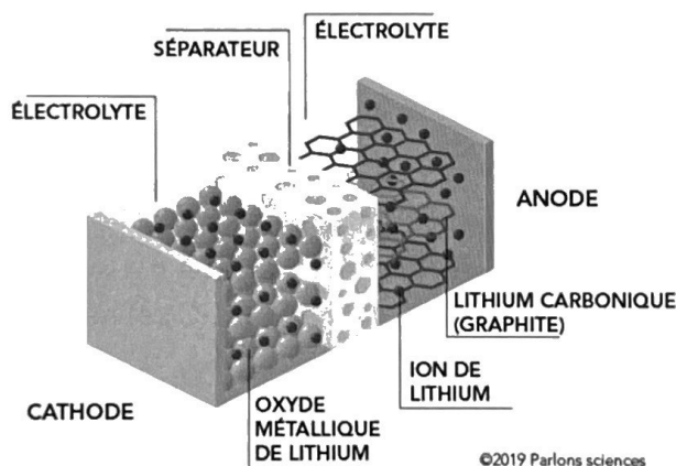
Figure 1 : Schéma d'une pile lithium-ion
