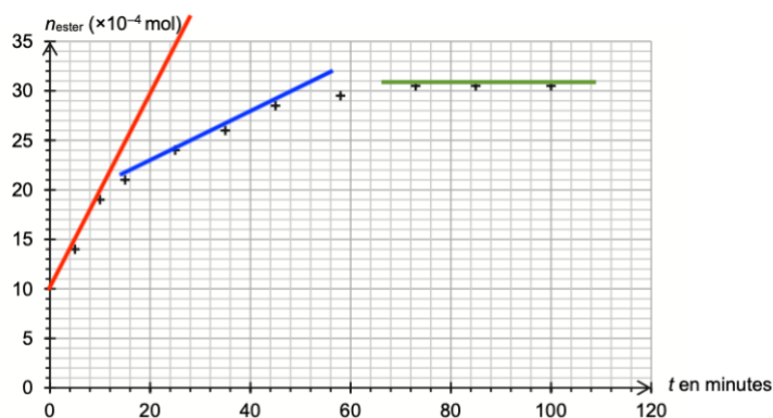
Figure 1. Courbe représentant l'évolution temporelle de n_{\text{ester}}
