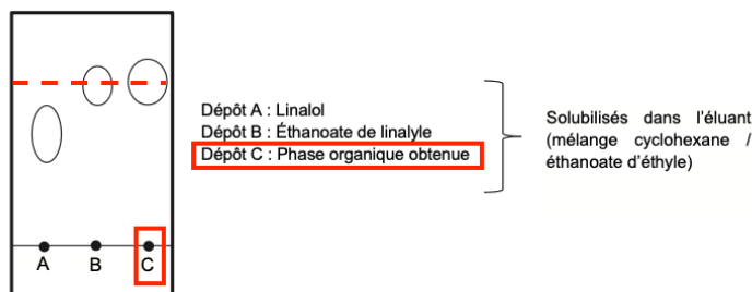
Figure 3. Chromatogramme obtenu expérimentalement après la deuxième synthèse
