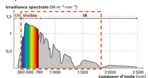
Document 4 – Spectre d'émission du Soleil
