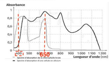
Document 3 – Spectres d'absorption
