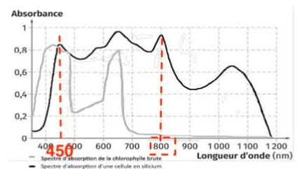
Document 3 – Spectres d'absorption
