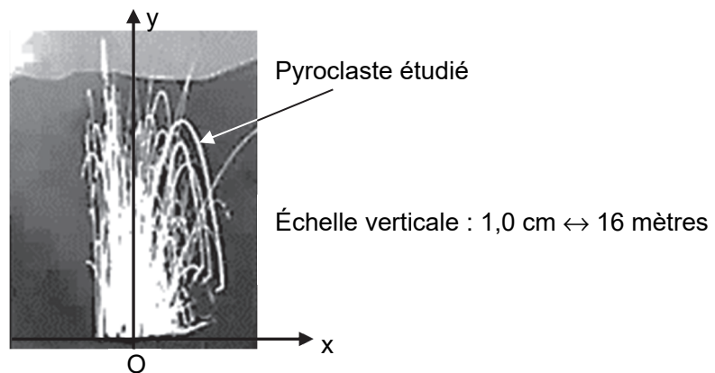
Figure 2. Photographie d'un événement explosif étudié en haut du mont Aso au Japon le 25 Avril 2015
