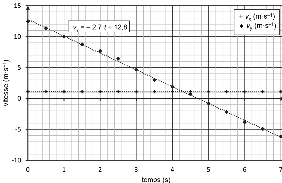
Figure 3. Évolution des coordonnées v_x et v_y du pyroclaste étudié lors de son mouvement
