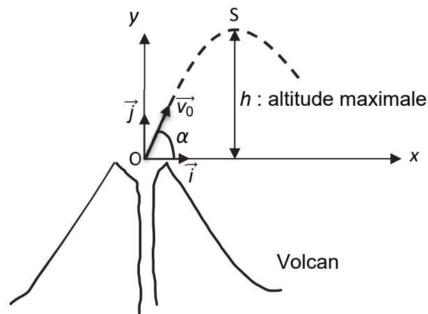
Figure 1. Représentation, sans souci d'échelle, de l'éjection du pyroclaste étudié lors d'une éruption volcanique
