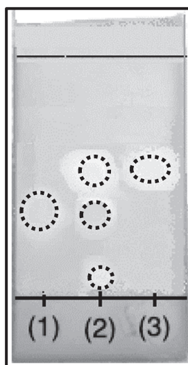
Figure 3. Chromatogramme obtenu
