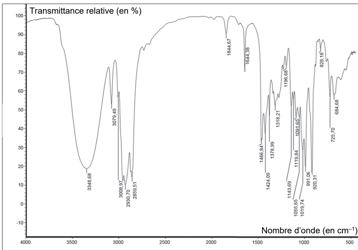
Figure 2. Spectre infrarouge du produit synthétisé
